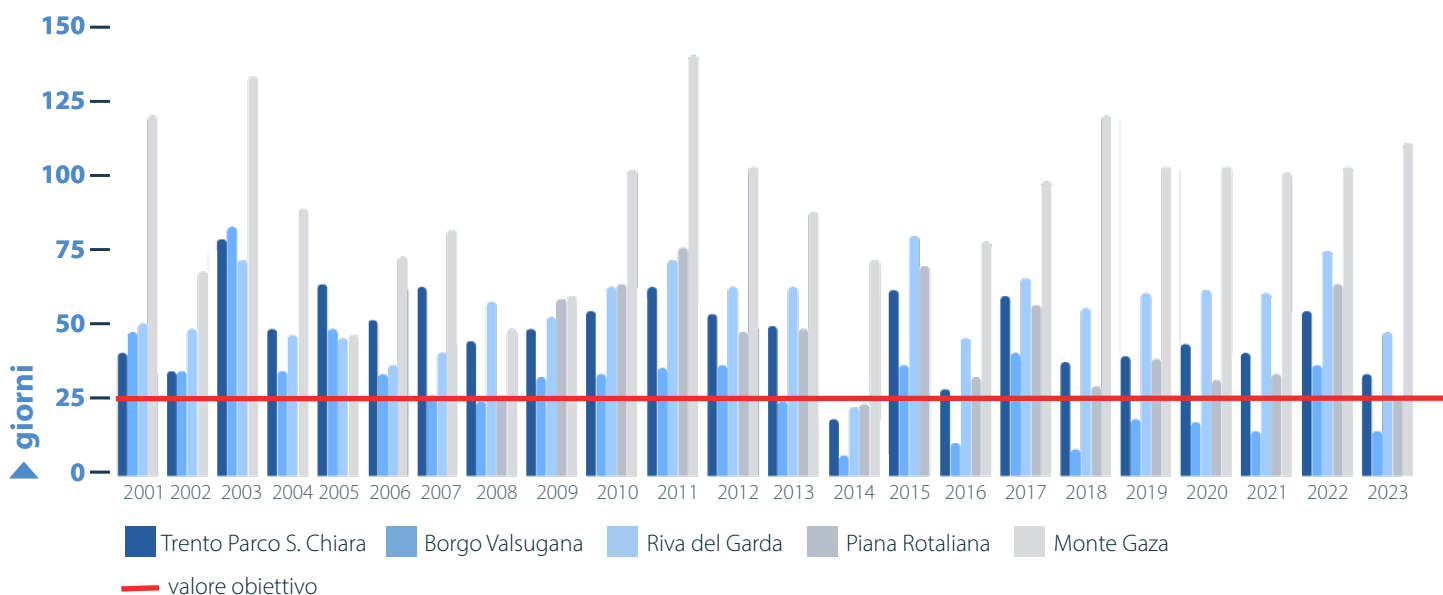
Figura 5.15: O 3 – superamenti del valore obiettivo
