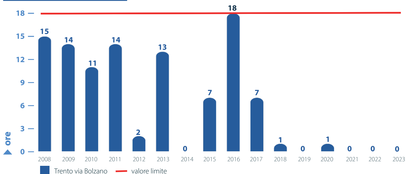
Figura 5.1: NO 2 – superamenti del valore limite orario
