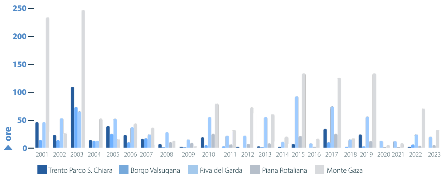
Figura 5.14: O 3 – superamenti della soglia di informazione
