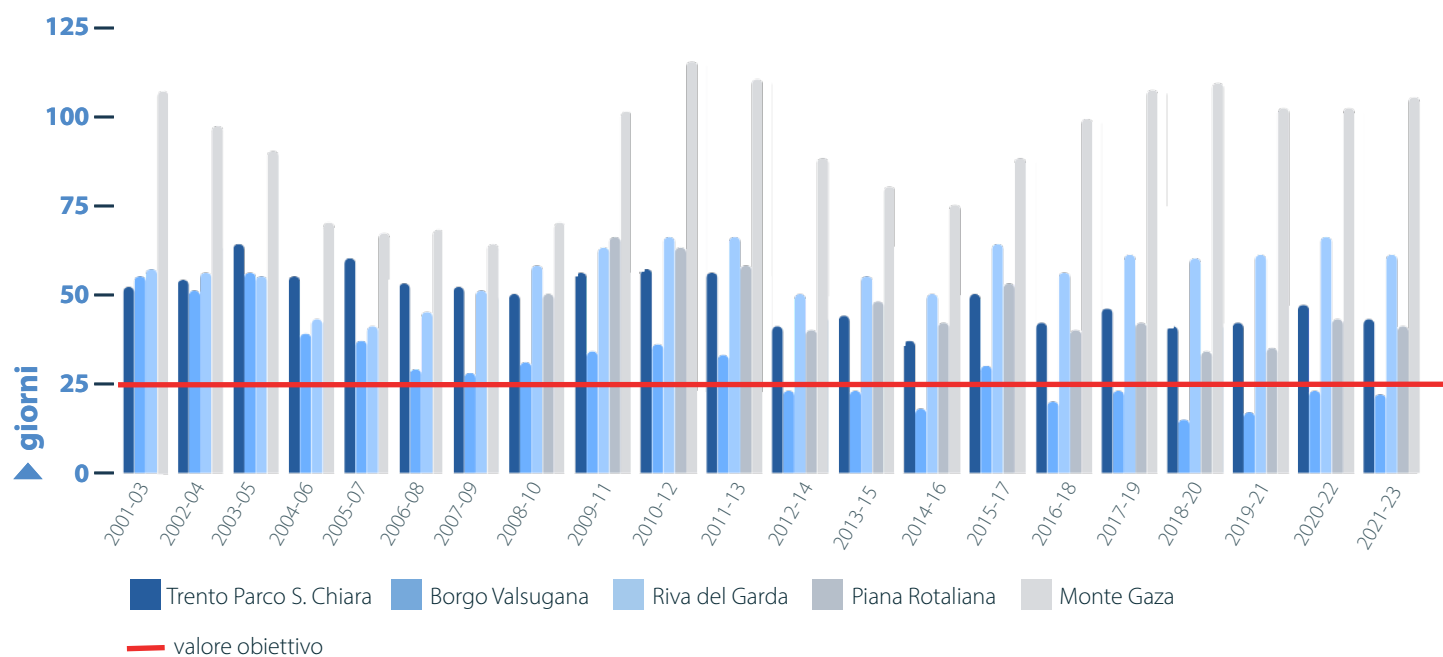
Figura 5.16: O 3 – superamenti del valore obiettivo, media su 3 anni
