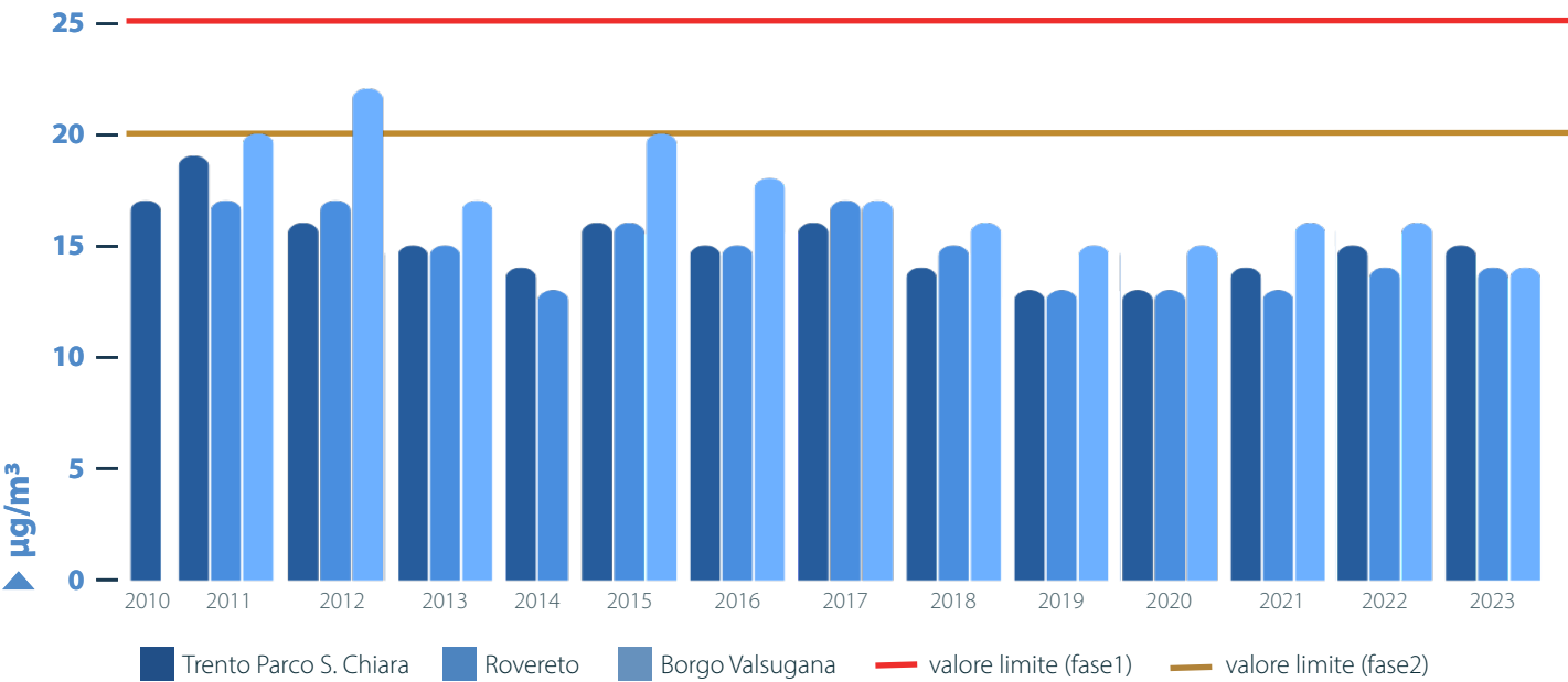
Figura 5.5: PM2,5 – media annua
